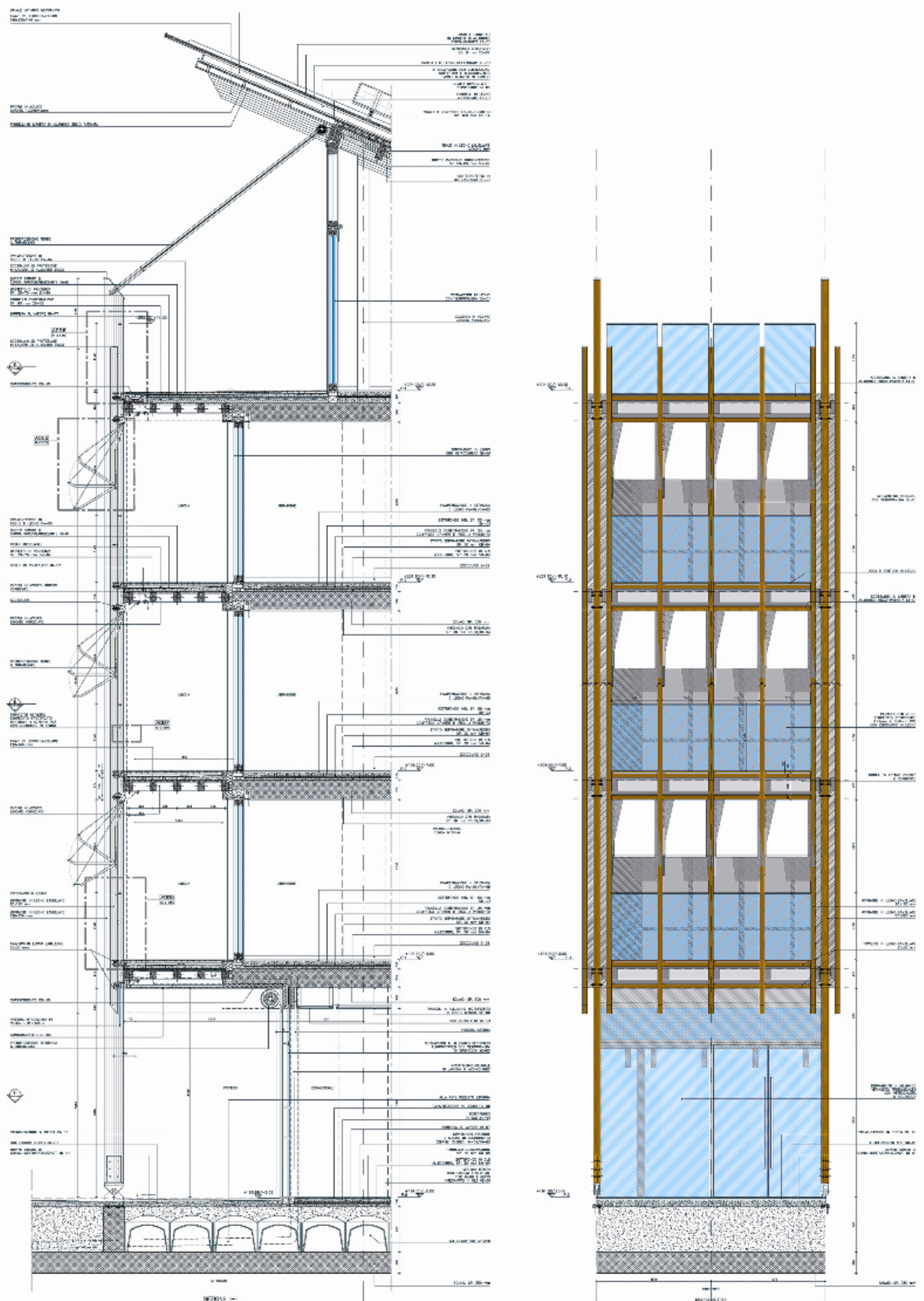
Fig.12: sezione di dettaglio delle residenze e degli uffici
